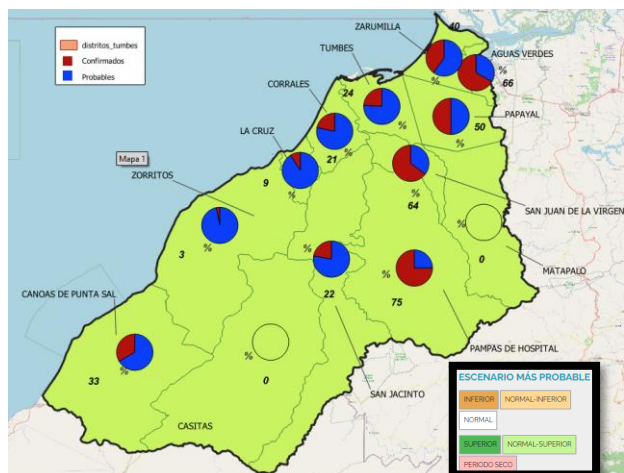
Gráfico 8. Pronóstico climático de precipitaciones y casos de dengue, Región de Tumbes, SE 01-08/2025
