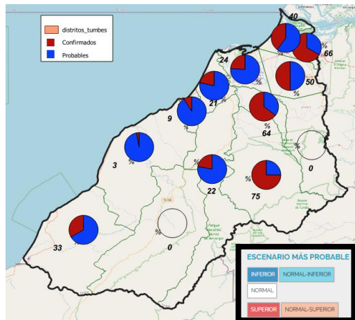
Gráfico 10. Pronóstico climático de temperatura mínima y casos de dengue, Región de Tumbes, SE 01-08/2025
