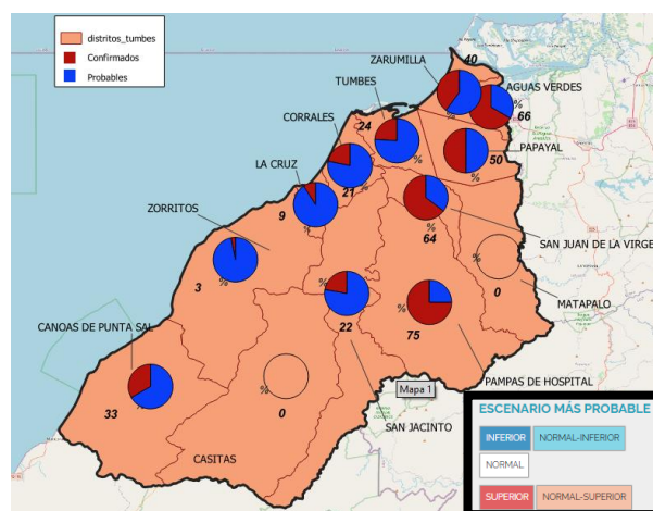
Gráfico 9. Pronóstico climático de temperatura máxima y casos de dengue, Región de Tumbes, SE 01-08/2025
