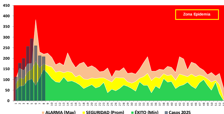
Gráfico 25. Comportamiento de las EDAs en población general, Región Tumbes, 2025 (SE01-08) Canal Endémico
