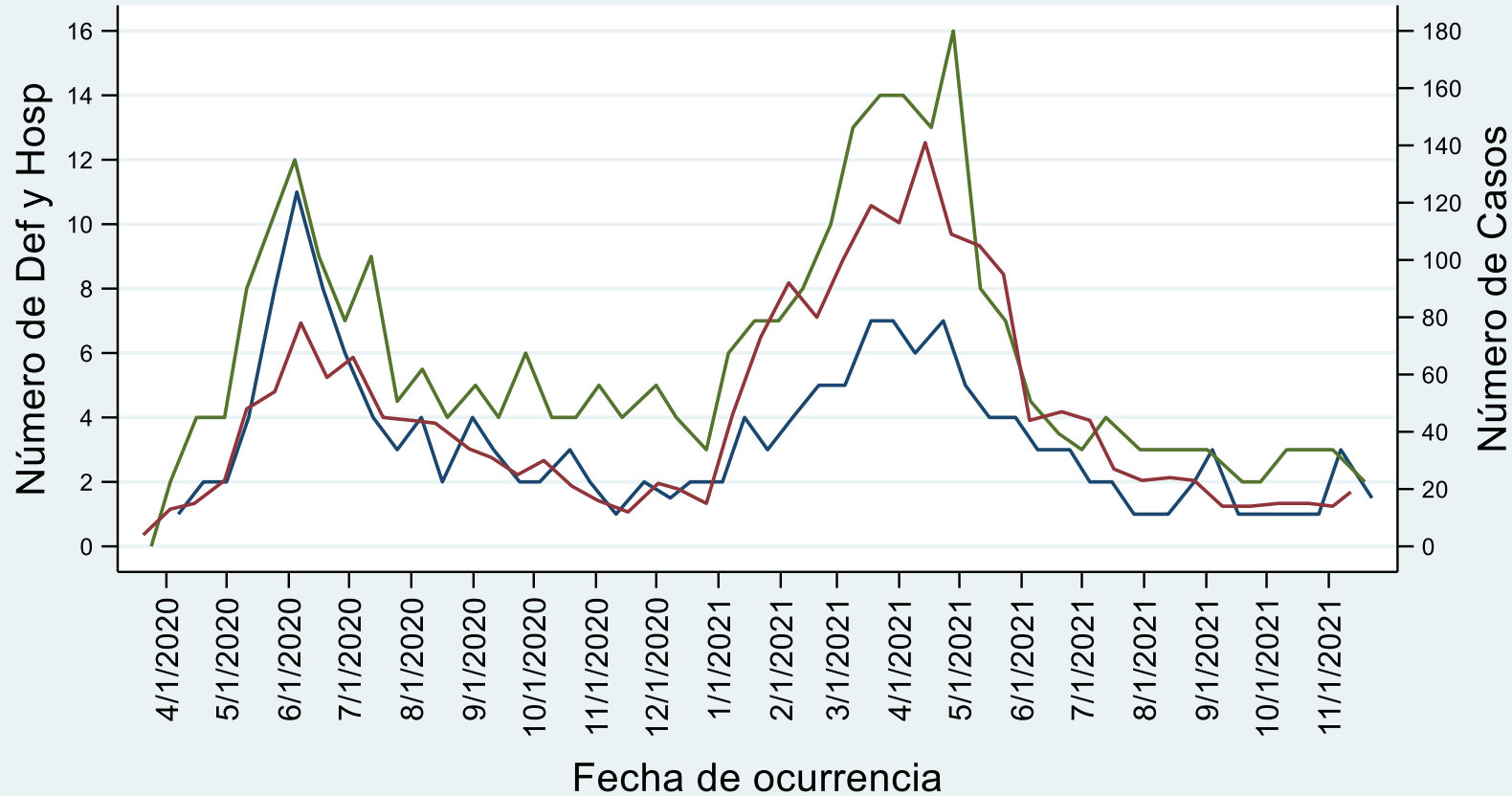
Comportamiento de la pandemia por COVID 19 Región de Tumbes al 24NOV21
