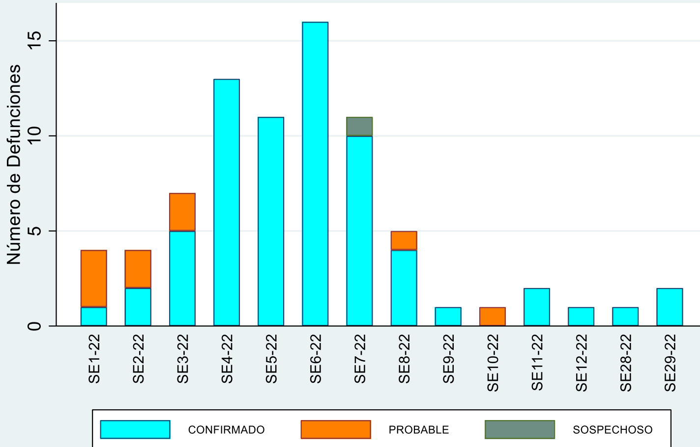
Defunciones por COVID19 según fecha de fallecimiento al 24/07/22
