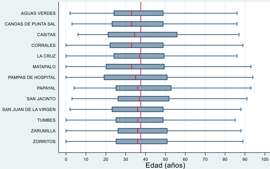
Comportamiento según edad y distritos de residencia DIRESA TUMBES al 240722
