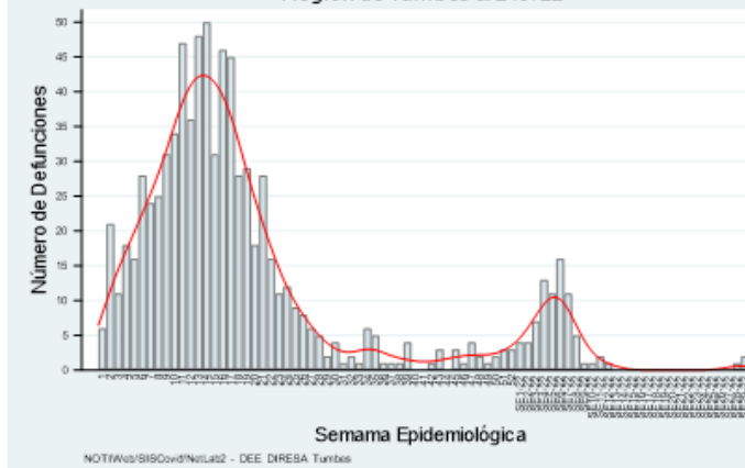
Defunciones por COVID19 Región de Tumbes al 24/07/2022
