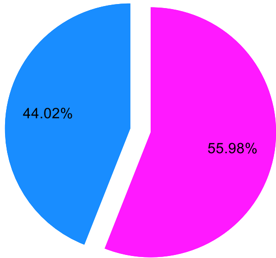
Casos de COVID19 por sexo Región Tumbes al 240722
