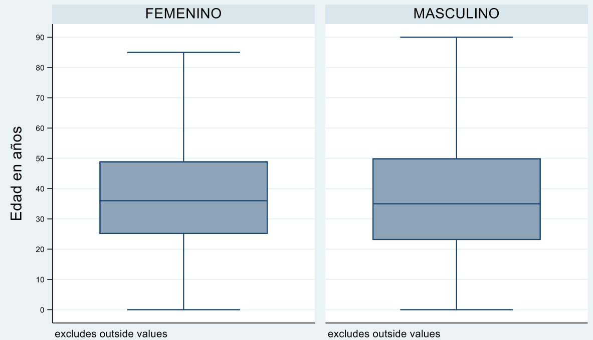
Distribución de casos según edad y sexo Región Tumbes al 240722
