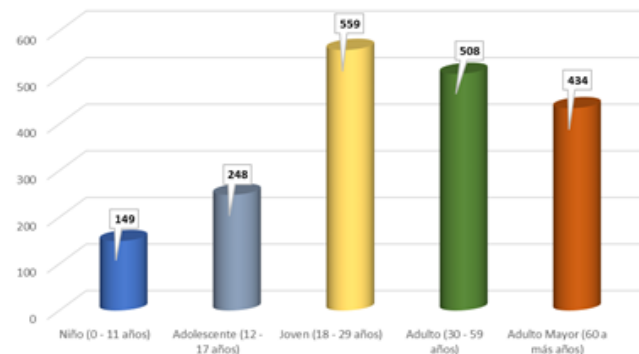
Defunciones por COVID19 Región de Tumbes al 24/07/2022
