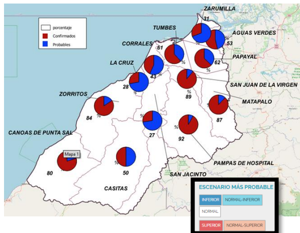
Gráfico 9. Pronóstico climático de temperatura mínima y casos de dengue, Región de Tumbes, SE 01-37/2025
