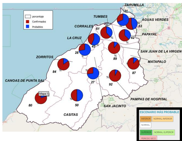
Gráfico 7. Pronóstico climático de precipitaciones y casos de dengue, Región de Tumbes, SE 01-37/2025
