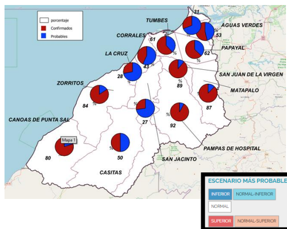
Gráfico 8. Pronóstico climático de temperatura máxima y casos de dengue, Región de Tumbes, SE 01-37/2025
