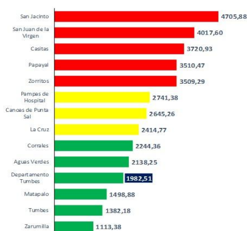
Gráfico 11. Incidencia acumulada distrital de IRAs en < de 5 años, Región Tumbes, 2026 (SE01-17)
