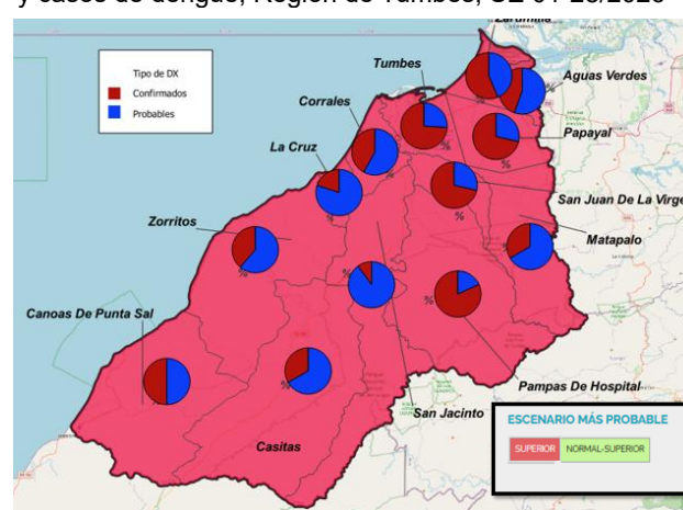
Gráfico 3. Pronóstico climático de temperatura máxima y casos de dengue, Región de Tumbes, SE 01-28/2026
