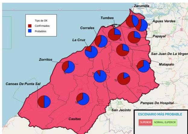
Gráfico 4. Pronóstico climático de temperatura mínima y casos de dengue, Región de Tumbes, SE 01-29/2026
