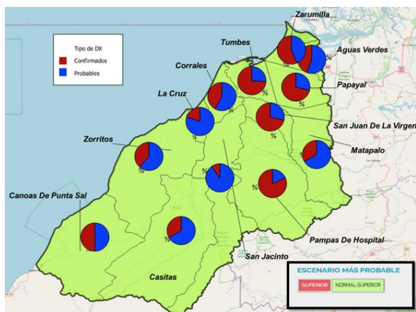
Gráfico 2. Pronóstico climático de precipitaciones y casos de dengue, Región de Tumbes, SE 01-29/2026
