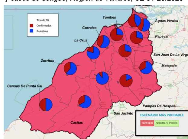
Gráfico 3. Pronóstico climático de temperatura máxima y casos de dengue, Región de Tumbes, SE 01-29/2026
